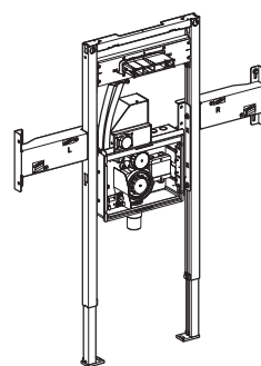
Modulo d'installazione per lavabo, parete altezza parziale.
